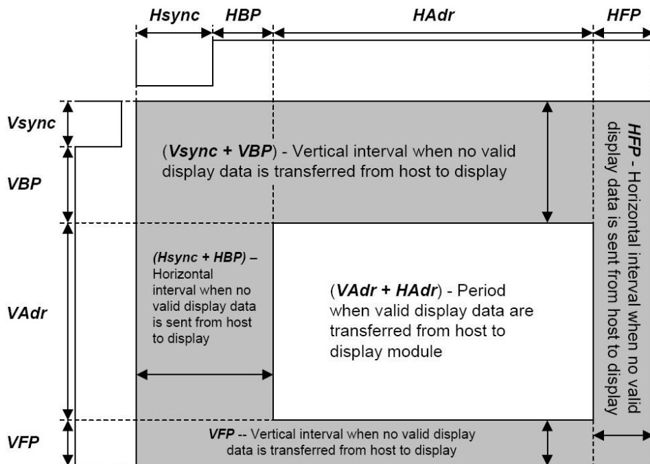
Figure 24. DPI Parameter
